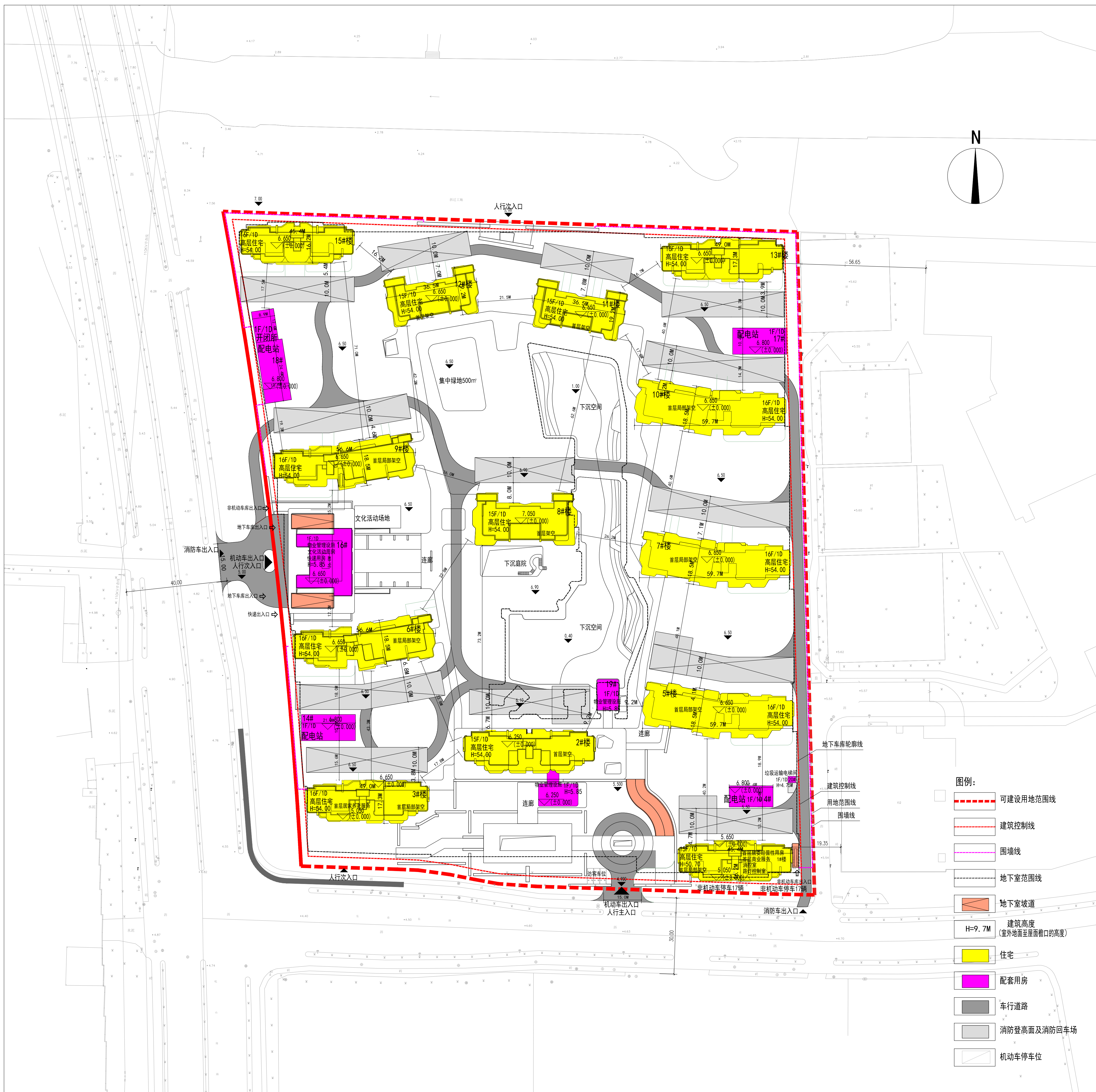
方案总平面图
