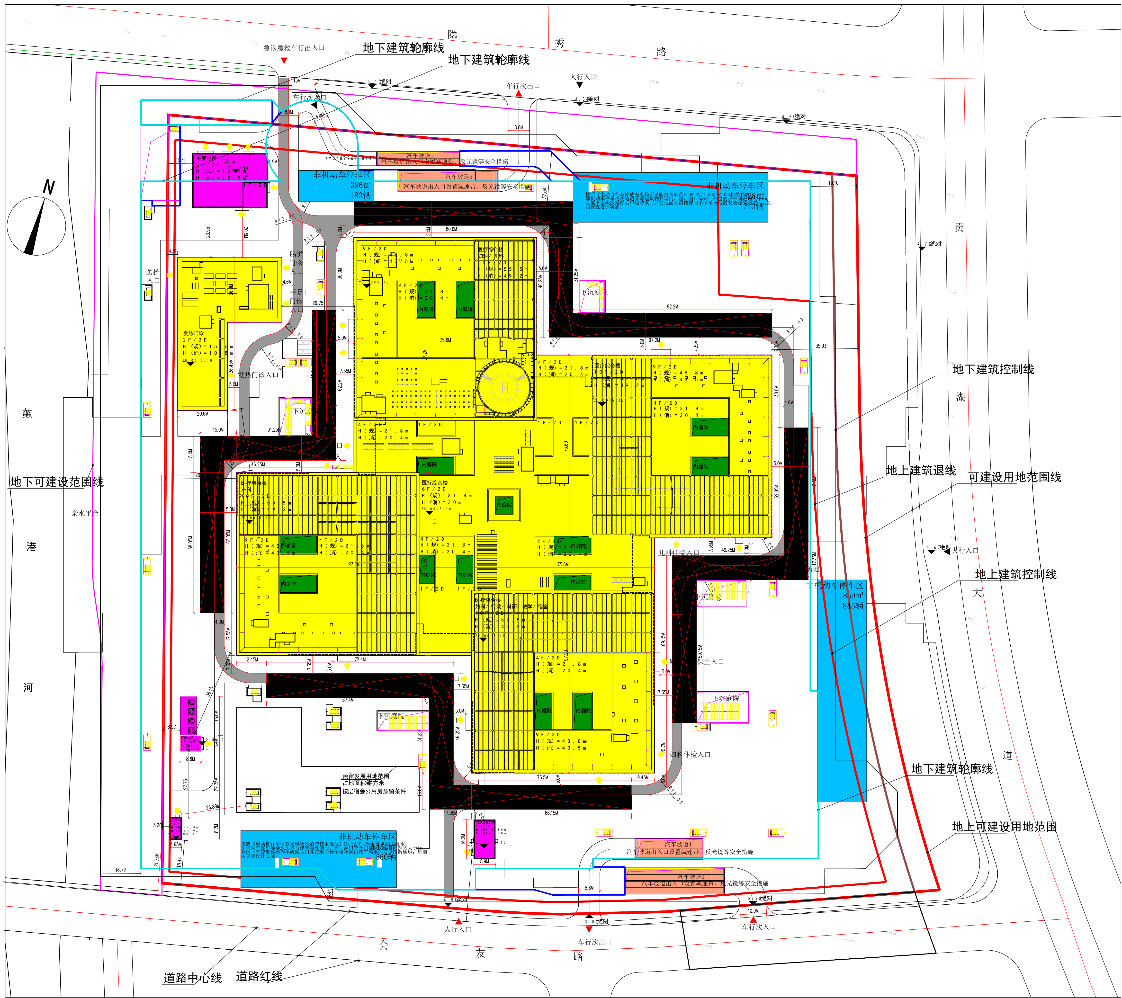
方案总平面图
